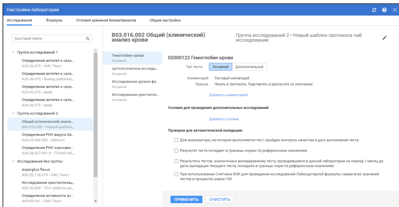
Рисунок 187 – Форма "Настройки лаборатории". Вкладка "Исследования"
