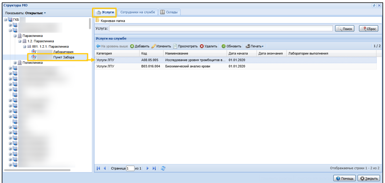
Рисунок 22 – Просмотр услуг для лабораторной службы
